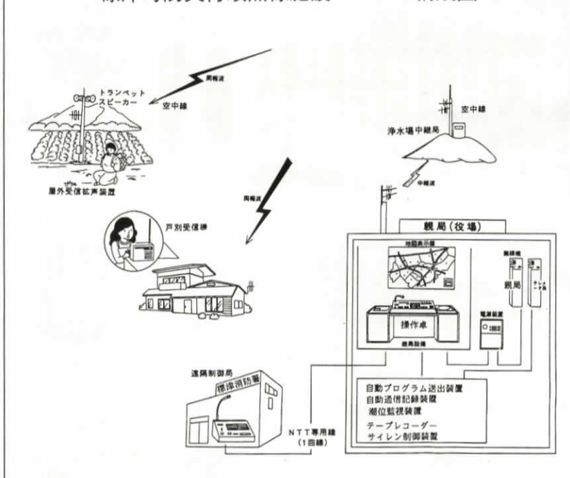
標津町防災行政無線施設システム構成図
