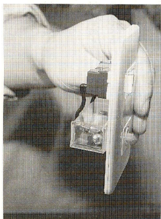
▲地震と同時に室内灯がつく「壁用スイッチボックス」も考案
