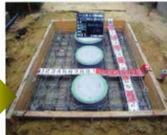
⑤上部スラブ配筋
