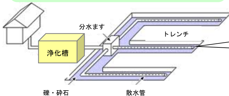
【浸透トレンチ設備施工例】
